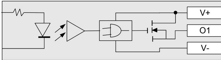
Fig. 3: Schema elettrico / Electric layout
